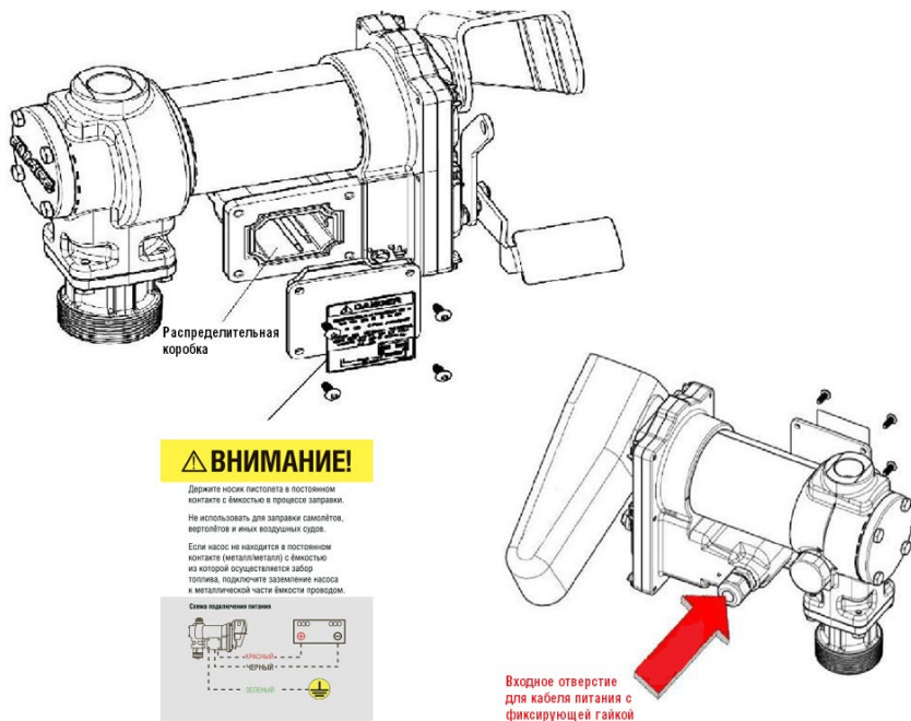
Рисунок 4. Схема мест для подключения питания
