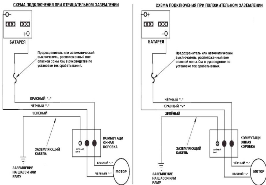
Рисунок 5. Принципиальная схема подключения питания
