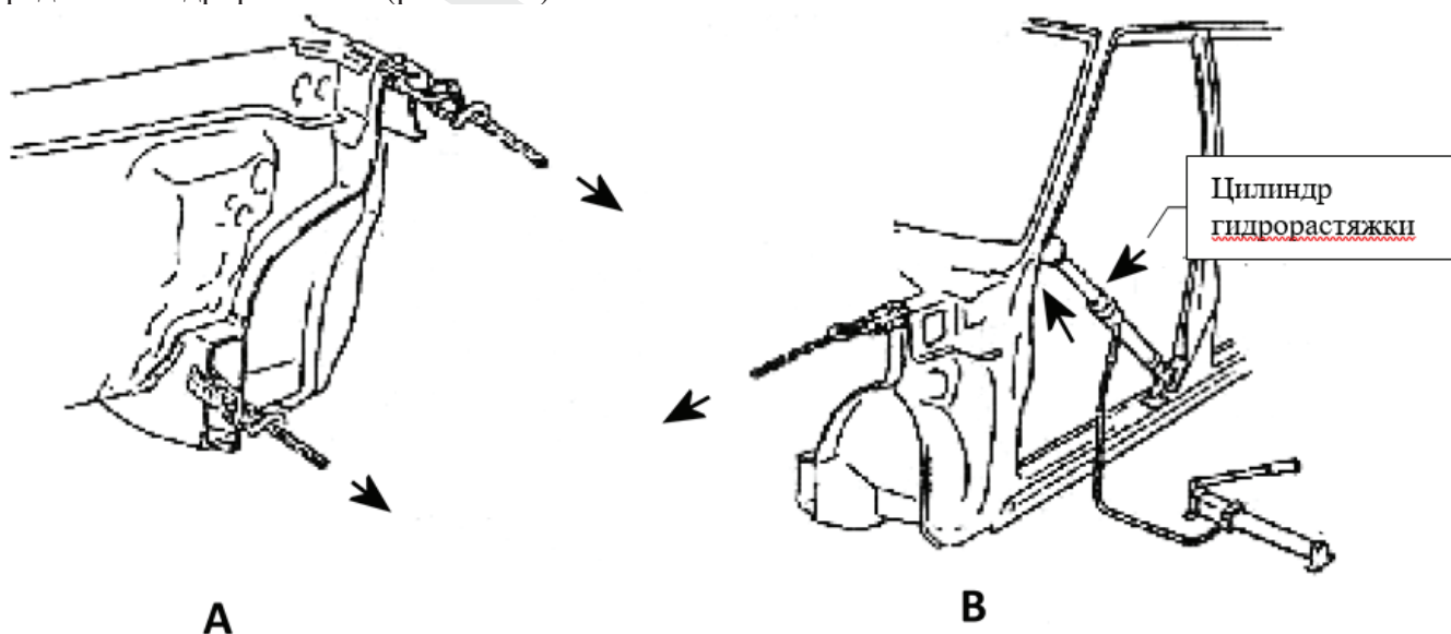
Рис. V-4 Восстановление передней стойки и передней скругленной панели
