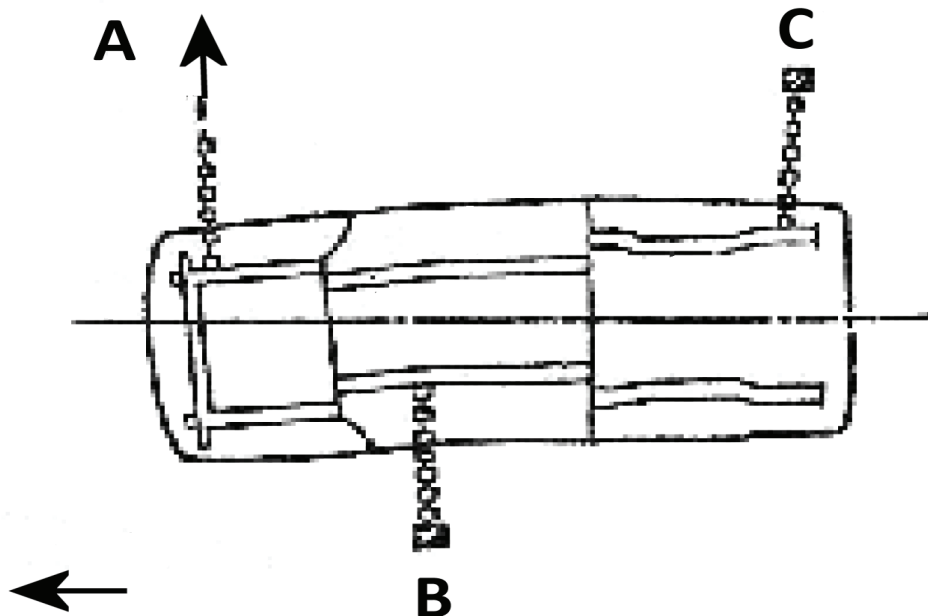
Рис. V-8 Исправление боковых вмятин от бокового удара по передней части автомобиля
