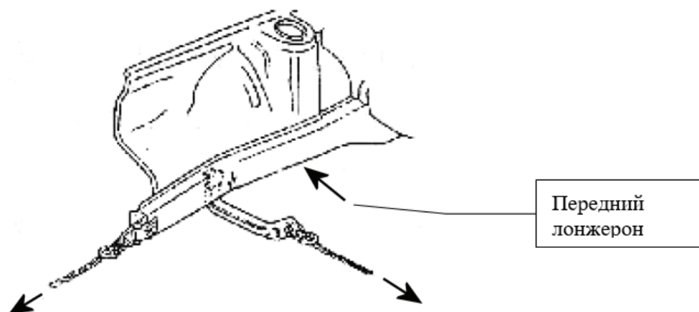
Рис. V-3 Восстановление бокового лонжерона
