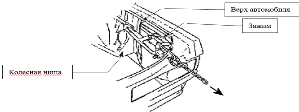
Рис. VI-1 Восстановление боковой вмятины в задней верхней части кузова
