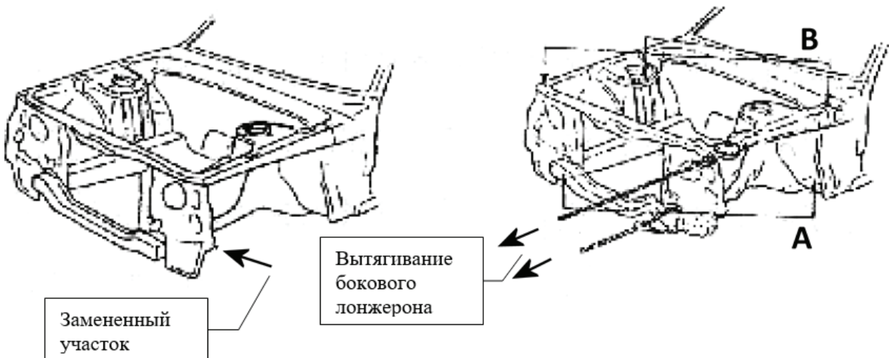
Рис. V-1 Восстановление передней панели части кузова
