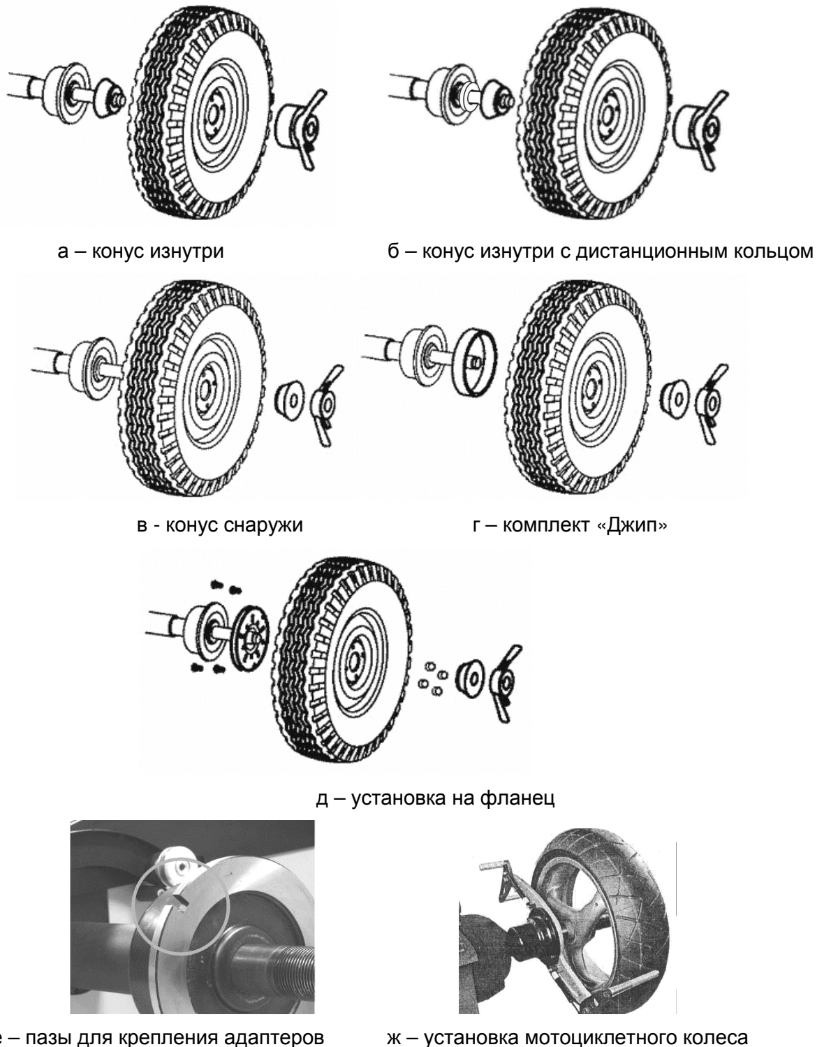
Рисунок 5.1 – Установка колеса
