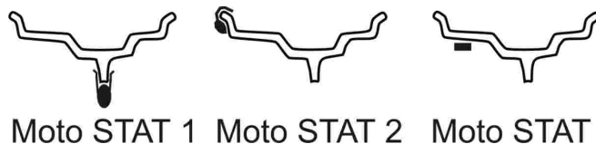
Рисунок 5.6 – Схемы установки грузов
