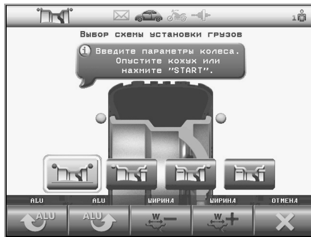
Рисунок 6.4 – Выбор схемы установки грузов
