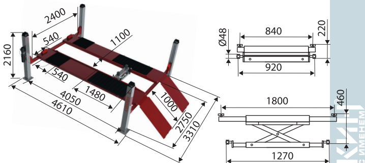
Рисунок 1 – Ямный домкрат
