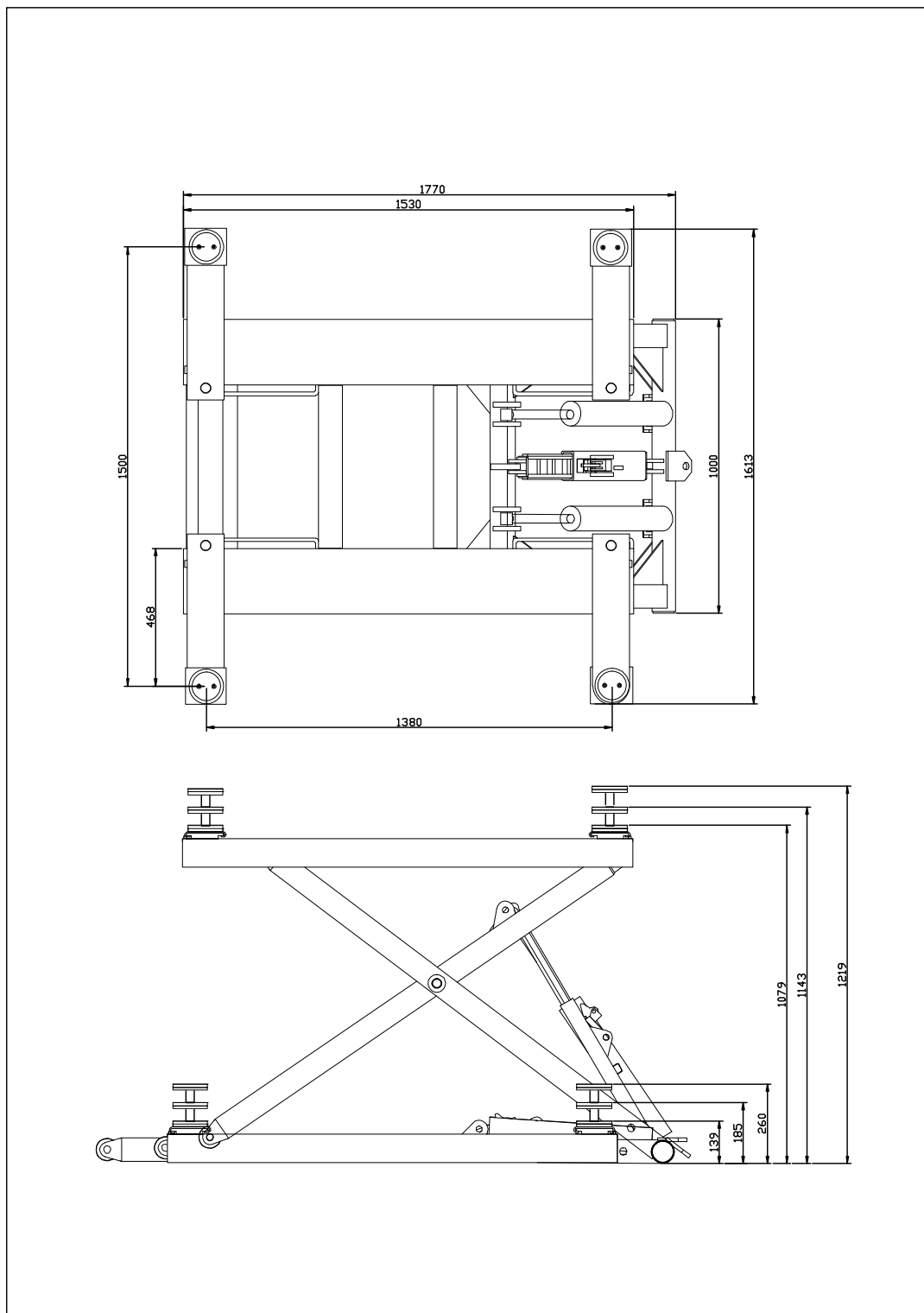
РИС. 2 - ЧЕРТЕЖ
