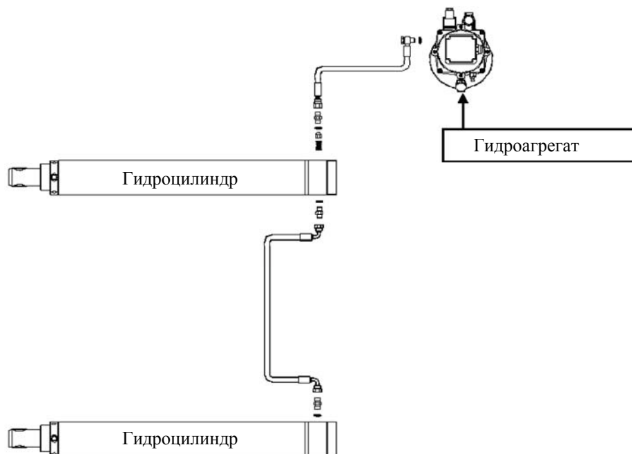
РИС. 5 – ГИДРАВЛИЧЕСКАЯ СИСТЕМА
