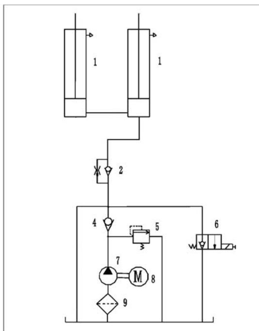
РИС. 5 – ГИДРАВЛИЧЕСКАЯ СИСТЕМА
