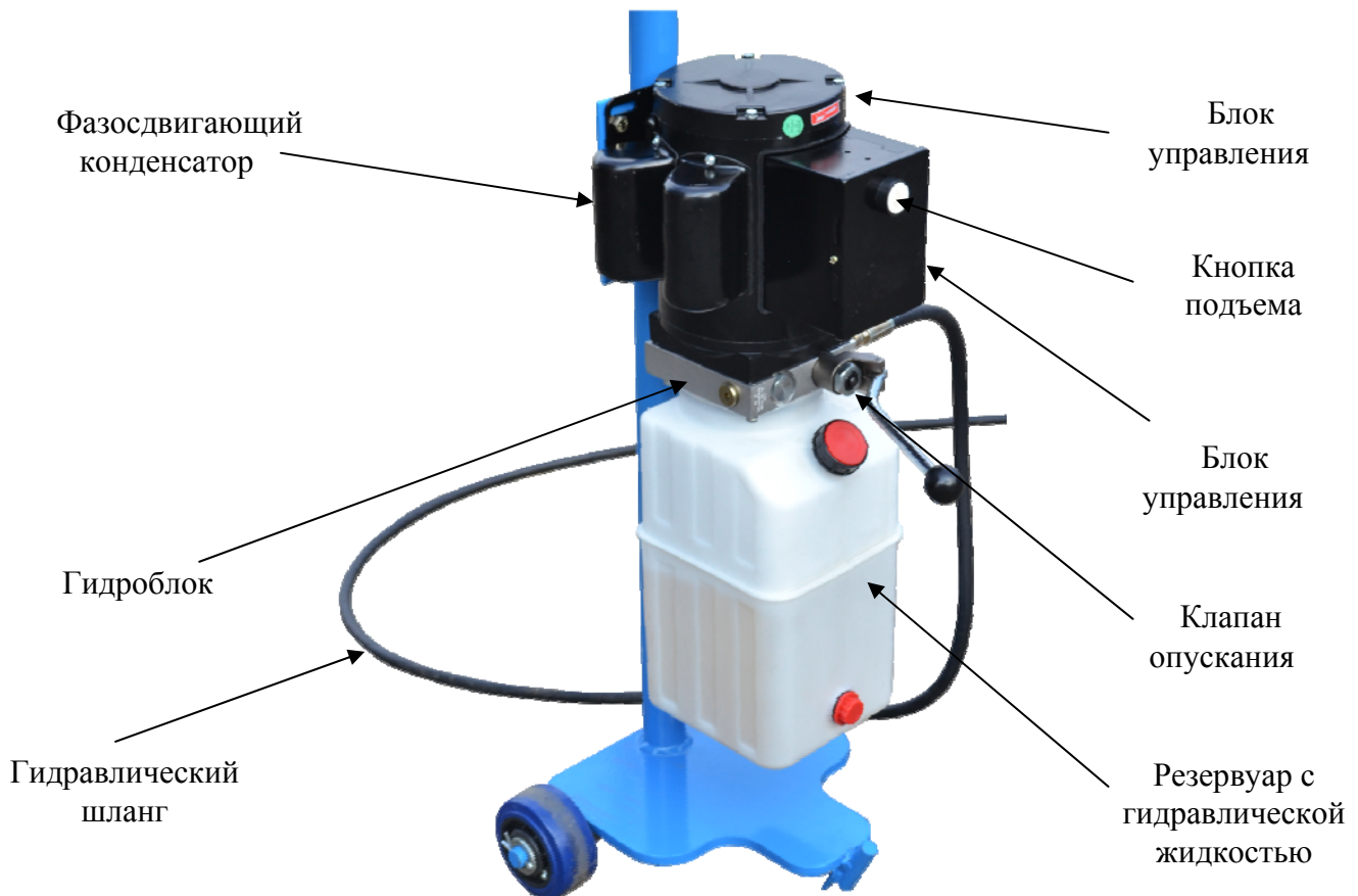
РИС. 3 - ГИДРАВЛИЧЕСКИЙ АГРЕГАТ
