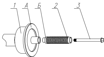
Рисунок 4.2 – Сборка вала
