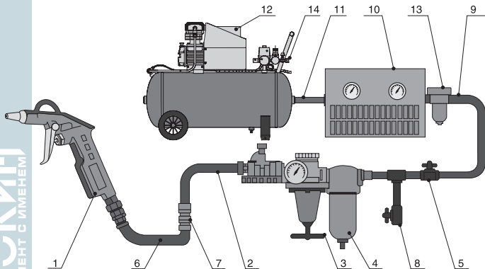
Рисунок 1 – Подключение пневматики
