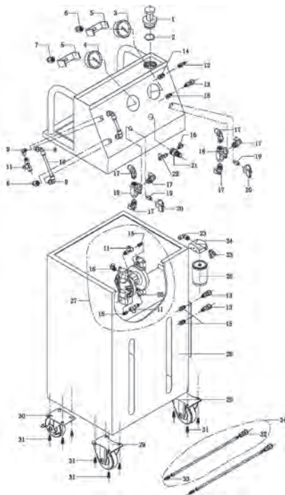
Рисунок 2 - Устройство изделия
